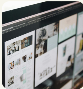
UX/UI
