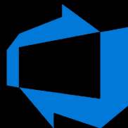
Azure DevOps
